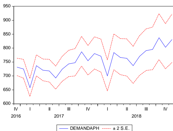
GRÁFICO 8: Pronóstico de la demanda de electricidad (en kwh) +/- dos errores estándar 2017-2018
