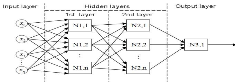
GRAFICA 5. MODELO DE UNA RED NEURONAL MULTICAPA
