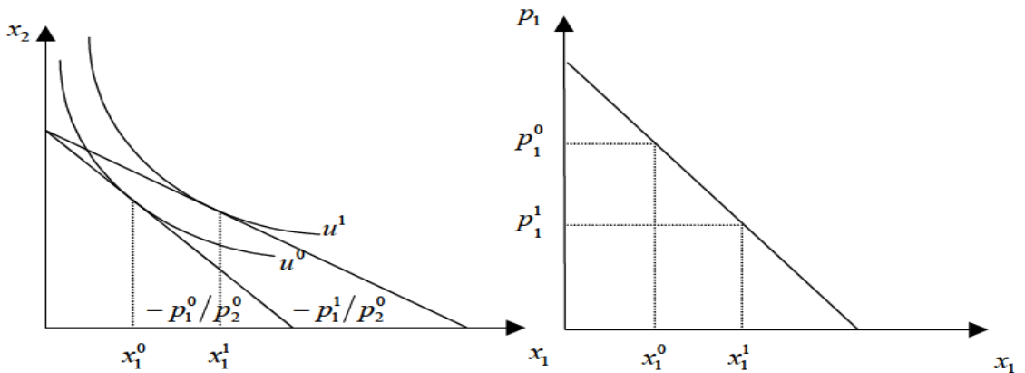
Gráfico 2: DERIVACIÓN DE LA DEMANDA ORDINARIA
