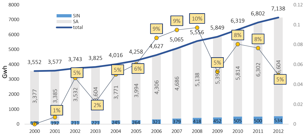
GRAFICO 3. EVOLUCIÓN DE LA DEMANDA DE ENERGÍA EN BOLIVIA (GWH) 2005 - 2012
